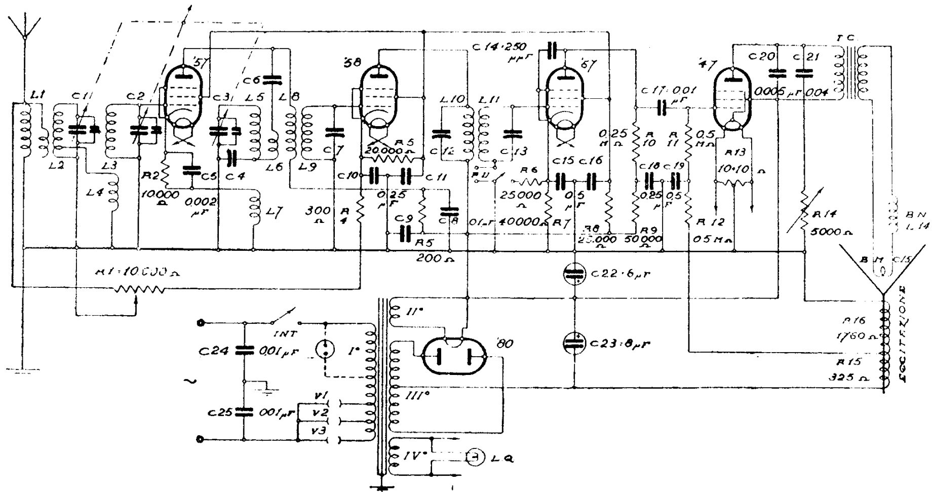
F.I.M.I. - MOD. PHONOLA «581» (ch. 560)
